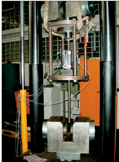
Abb. 12: Versuchseinrichtung zur Prüfung der Endverankerung
