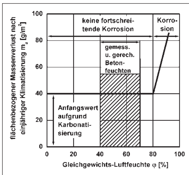
Abb. 5: Schematische Darstellung der Korrosionshemmung in Betonsandwichenelementen durch Austrocknung der Betonschale unter 80 % r.F. aufgrund außenseitig aufgebrachtener Wärmedämmung [11].
