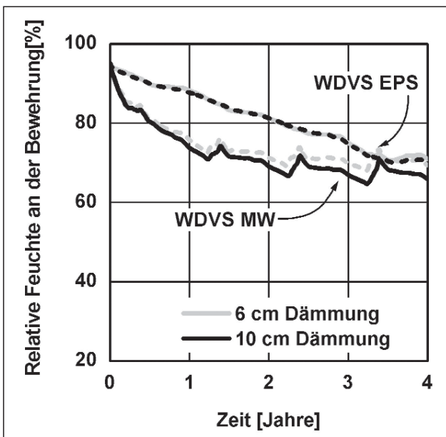
Abb. 7: Zeitliche Verläufe der relativen Feuchte an der Vorsatzschalenbewehrung der Dreischichtplatte aus Abb. 6 nach dem Aufbringen unterschiedlicher Außendämmsysteme mit 60 mm und 100 mm dicker Zusatzdämmung.
