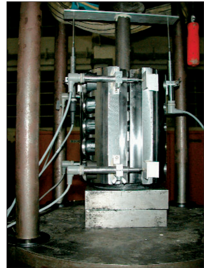
Abb. 13: Detail Verankerungskörper
