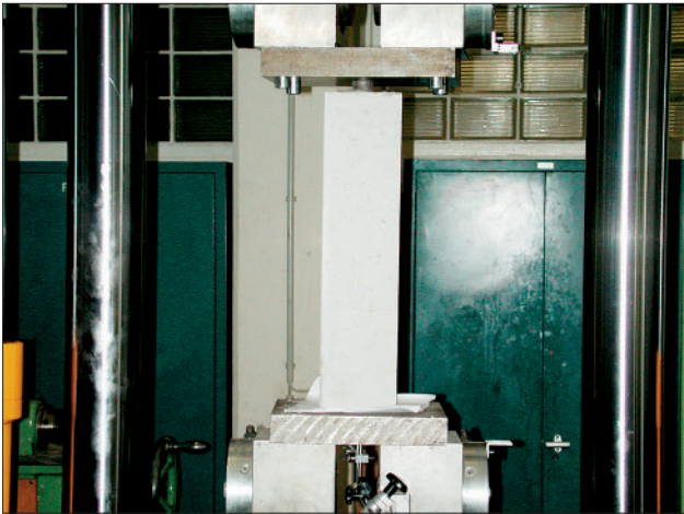
Abb. 15: Versuchsaufbau Push-in-Versuche
