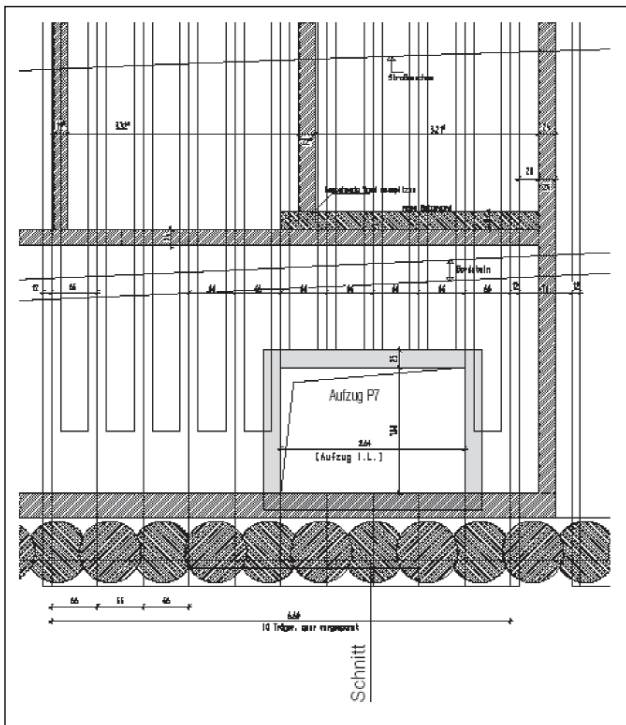
Abb. 9: Ansicht des Grundrisses des geplanten nachtraglichen Einbaus des Aufzuges
